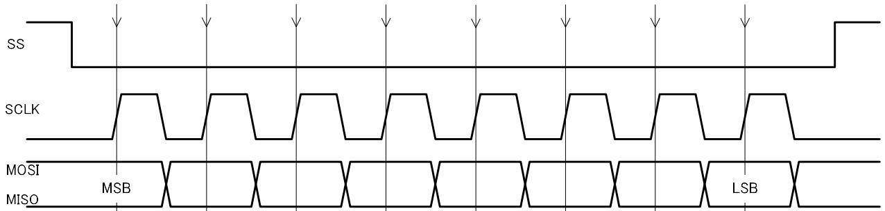
図 4.2.2.2 モード0、正パルス、前縁ラッチ、後端シフトのタイミング図
