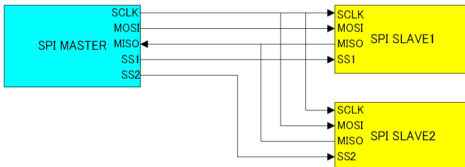
図 4.2.2.1 SPI 接続図
