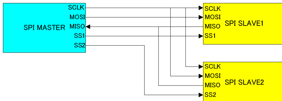
図 4.2.2.1 SPI 接続図
