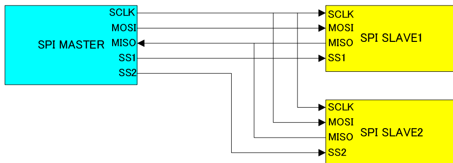
図 4.2.2.1 SPI 接続図
