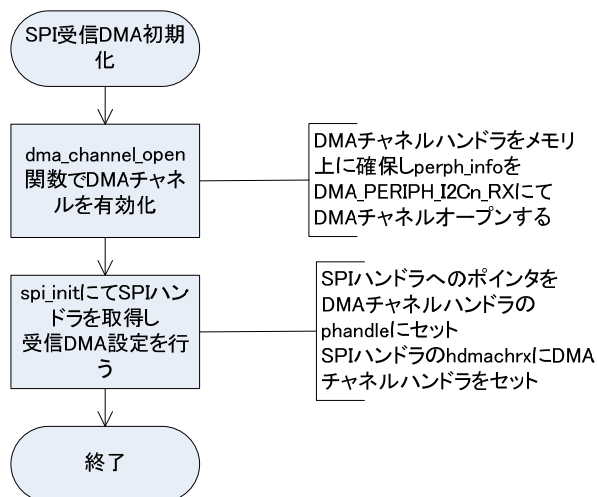
図 4.1.4.3.1 SPI-DMA 初期化
