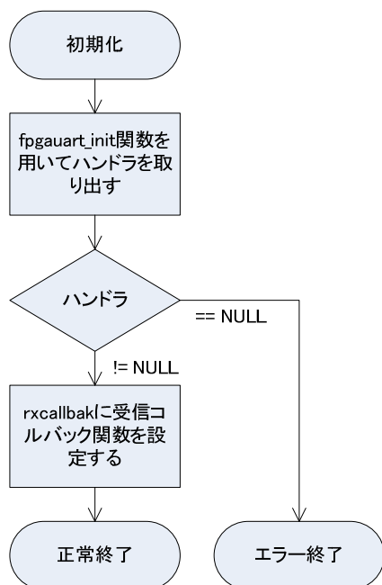
図 4.3.3.3.1 初期化
