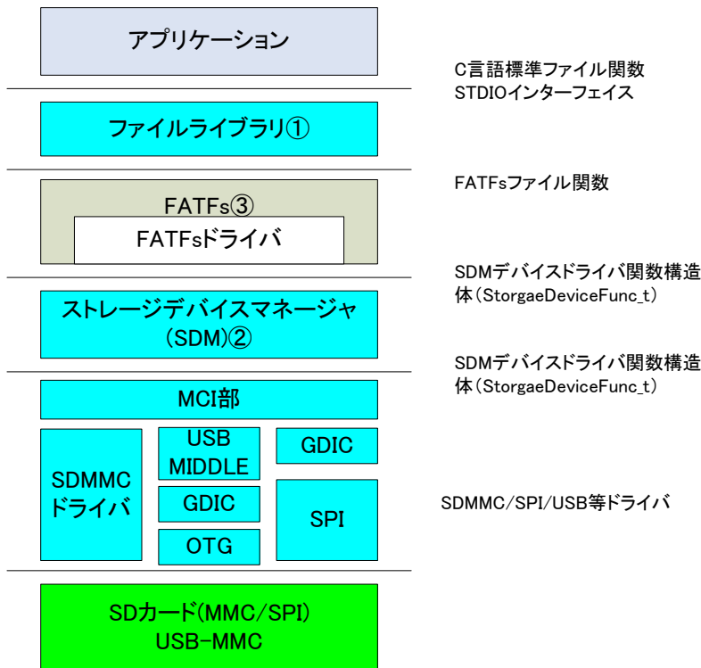
図 6.2.1 ファイルシステムのレイヤ構造
